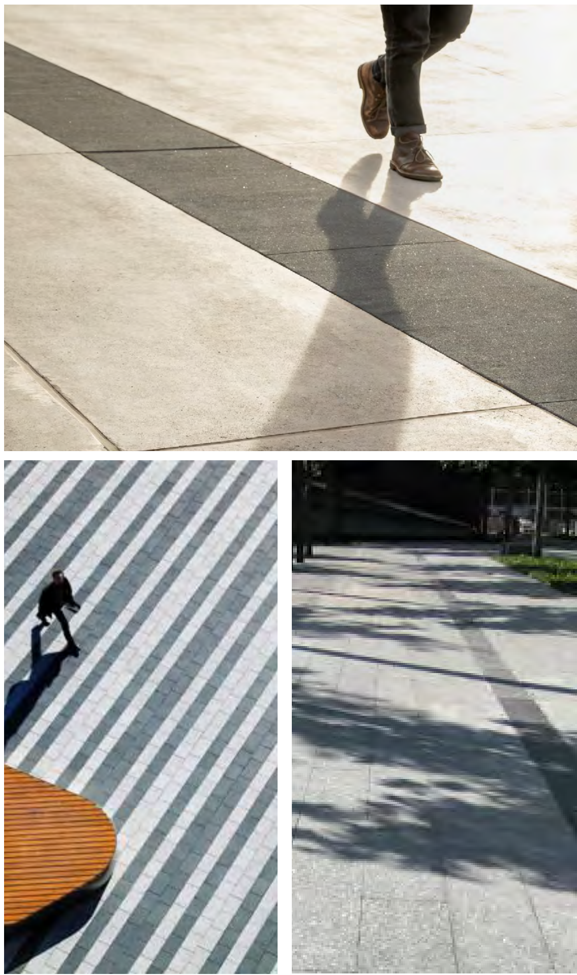
LINEAR MOMENTUM
